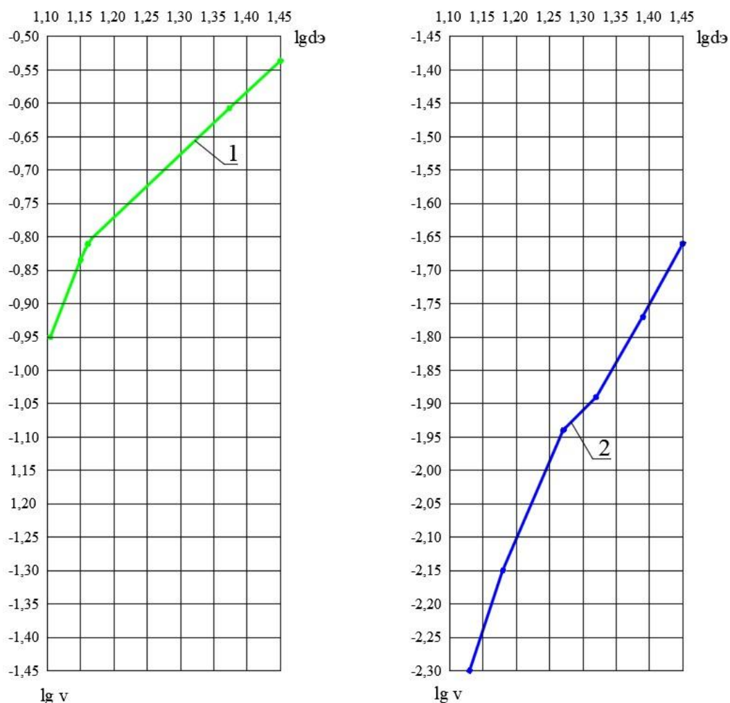
Рис. 8. График зависимости скорости осаждения частиц от их размера выраженная через логарифмическую функцию: 1 – логарифмическая кривая скорости осаждения, построенная по результатам натурных исследований; 2 – логарифмическая кривая скорости осаждения, определенная с помощью закона Стокса.
