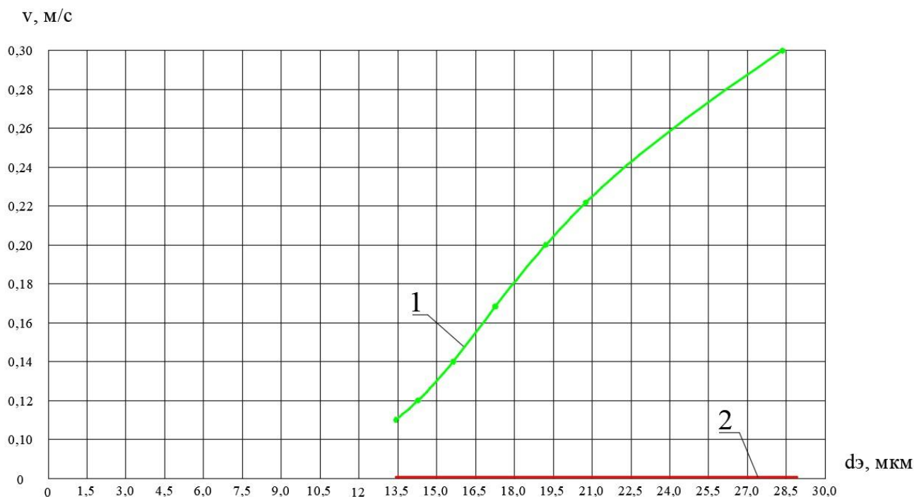
Рис. 7. – График зависимости скорости осаждения частиц от их размера:
