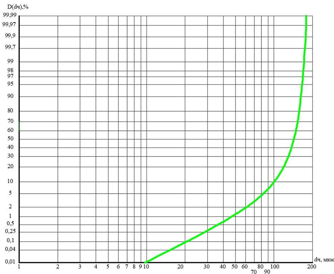
Рис. 3. – Усредненный интегральный график дисперсного состава пыли
